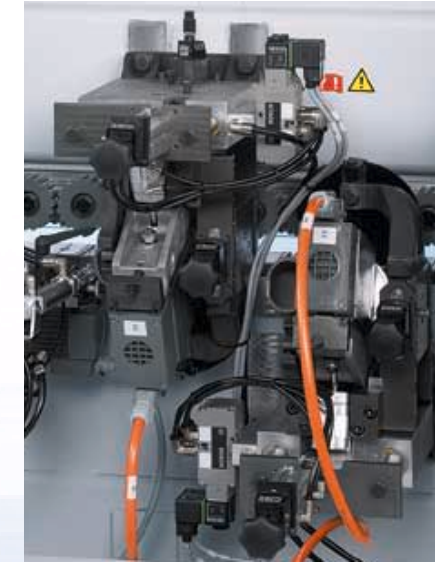
Fräsaggregat Multifunktionales Fräsaggregat mit DFC-Werkzeugtechnologie für optimale Absaugung.
